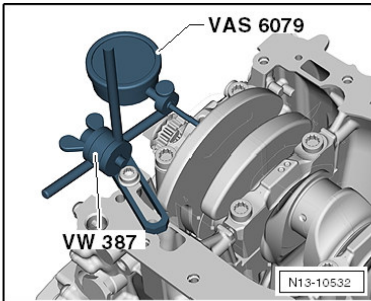
Fig. 19: Identifying VAS 6079 & VW 387
