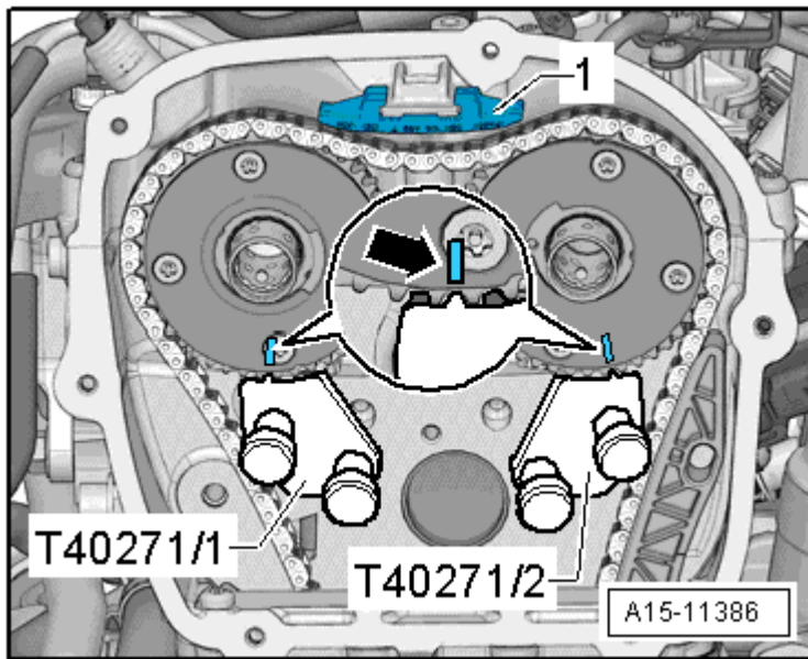
Fig. 119: Mark The Camshaft Sprocket
